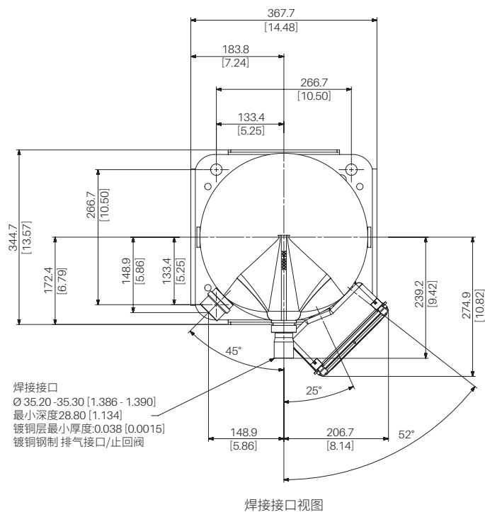
焊接接口视图
