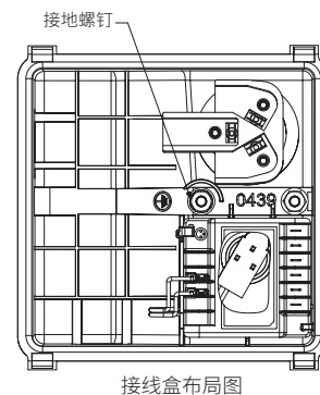
接线盒布局图
