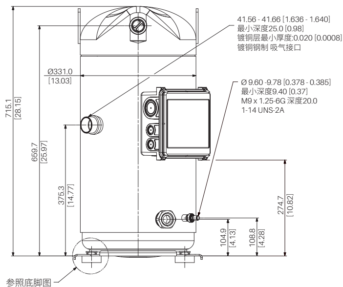
参照底脚图
