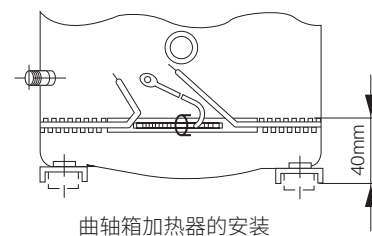
曲轴箱加热器的安装
