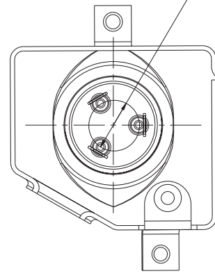
接线盒布置 2:1
