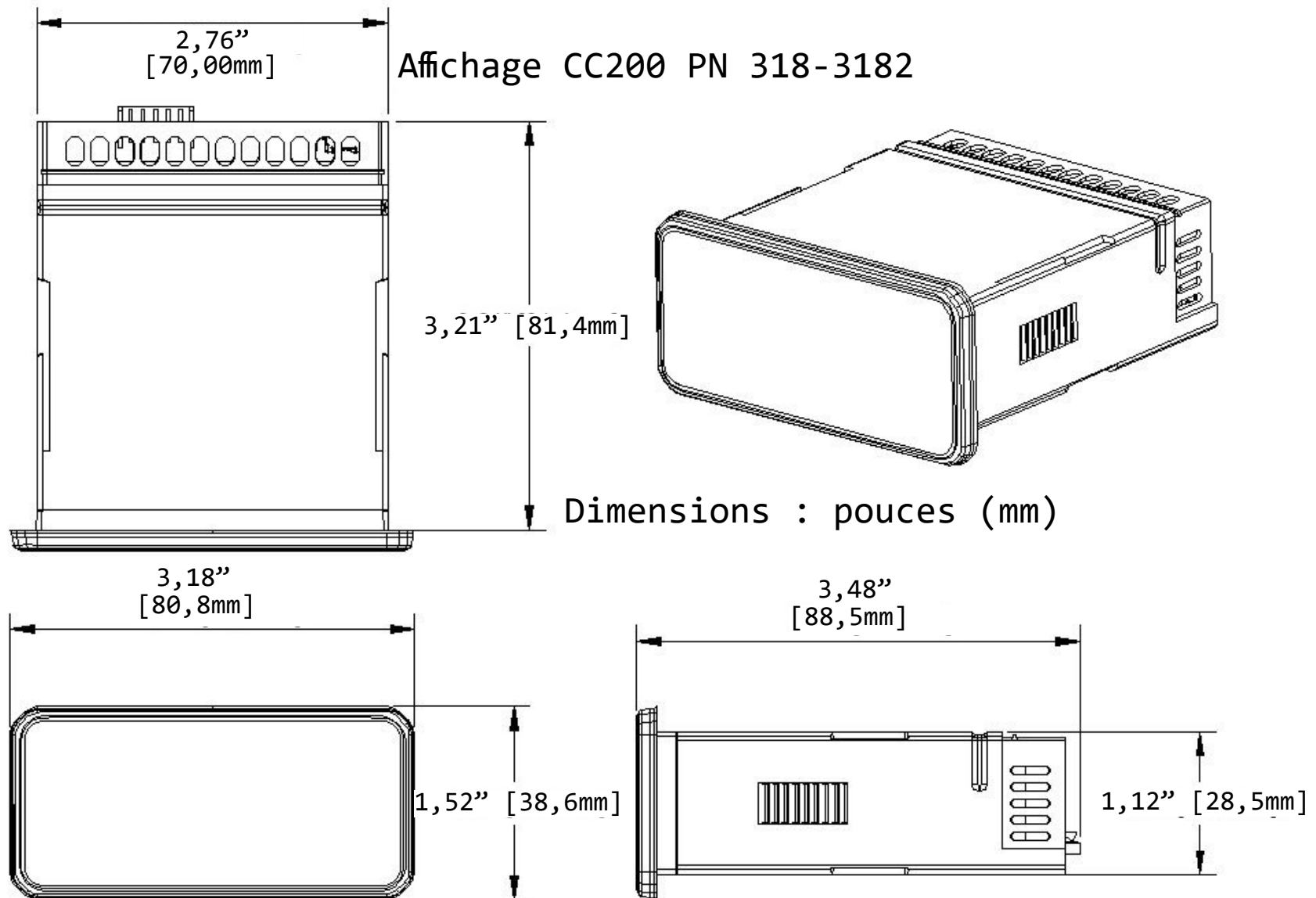
Dimensions de l'affichage CC200 P/N 318-3182
