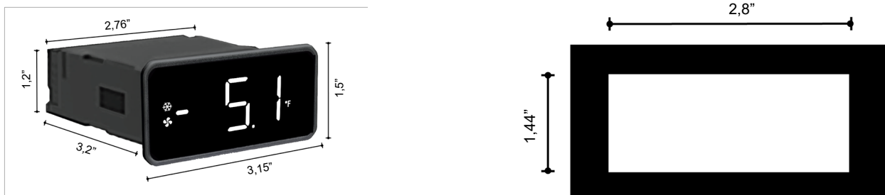
Dimensions de l'affichage du boîtier CC200
