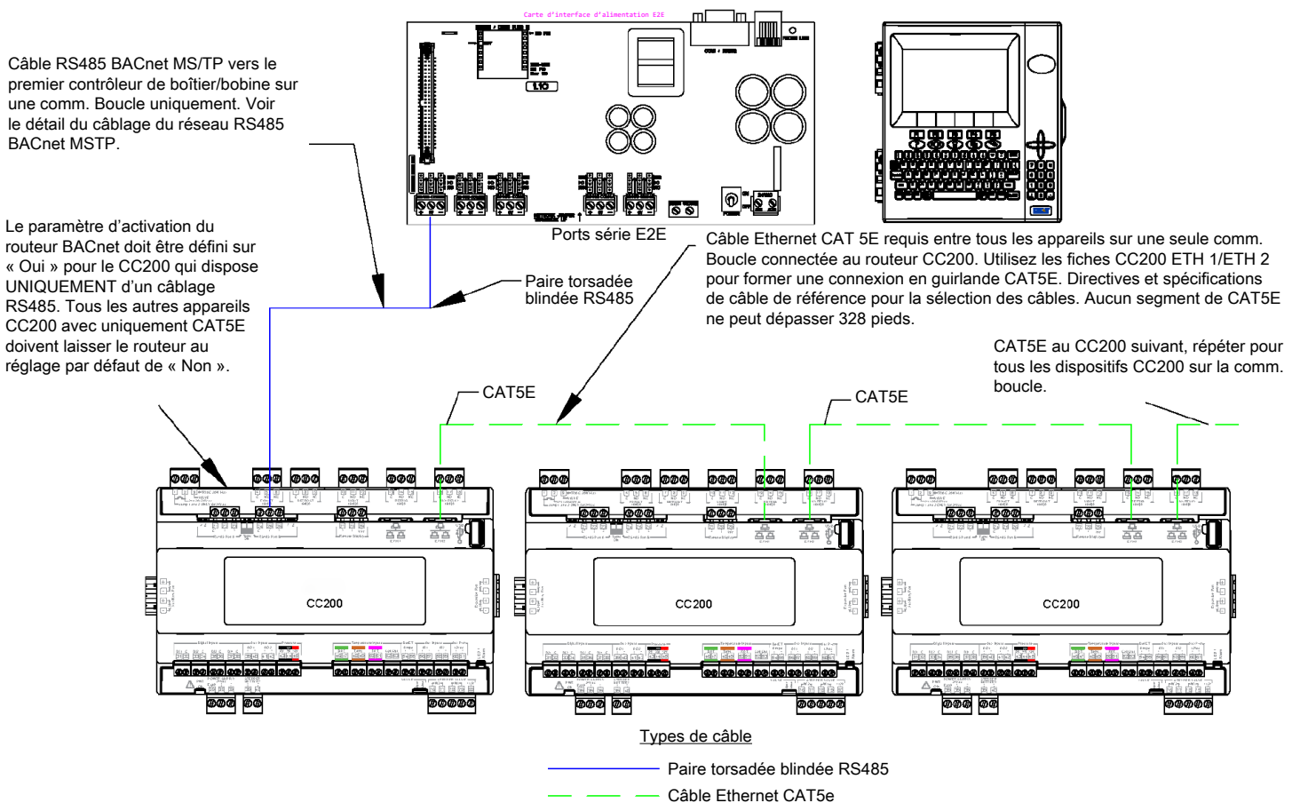
Présentation de la topologie du réseau
