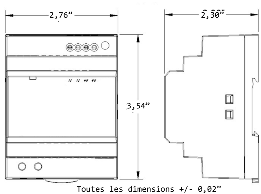
Dimensions de l'alimentation 92 watts P/N 318-3184
