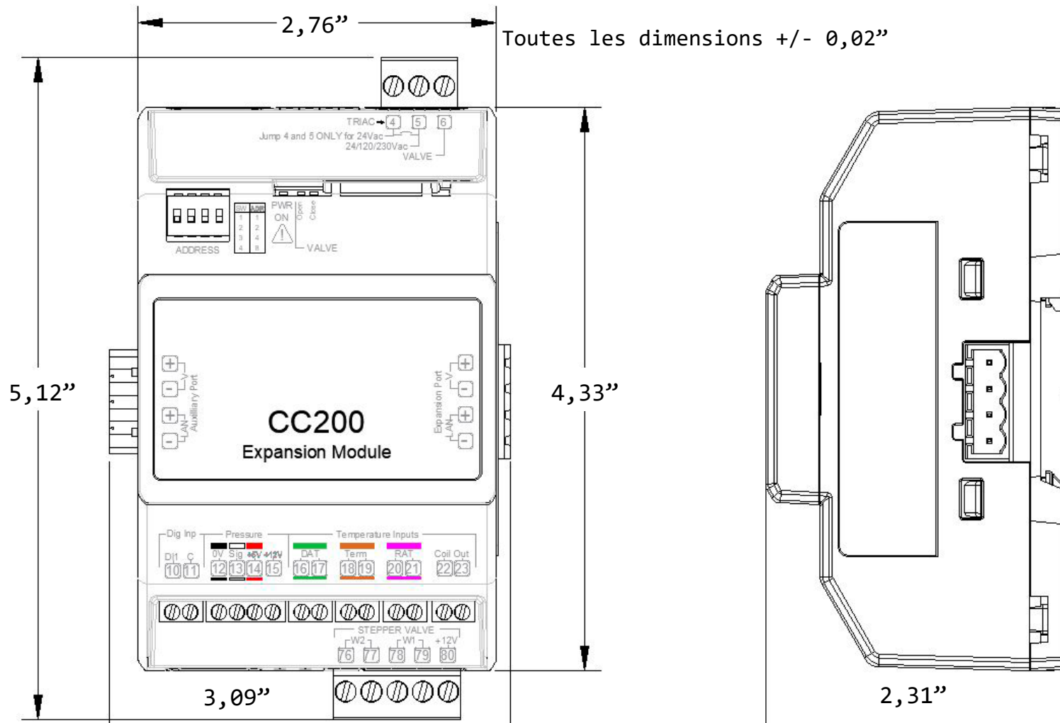
Dimensions du module d'extension CC200 P/N 318-3181
