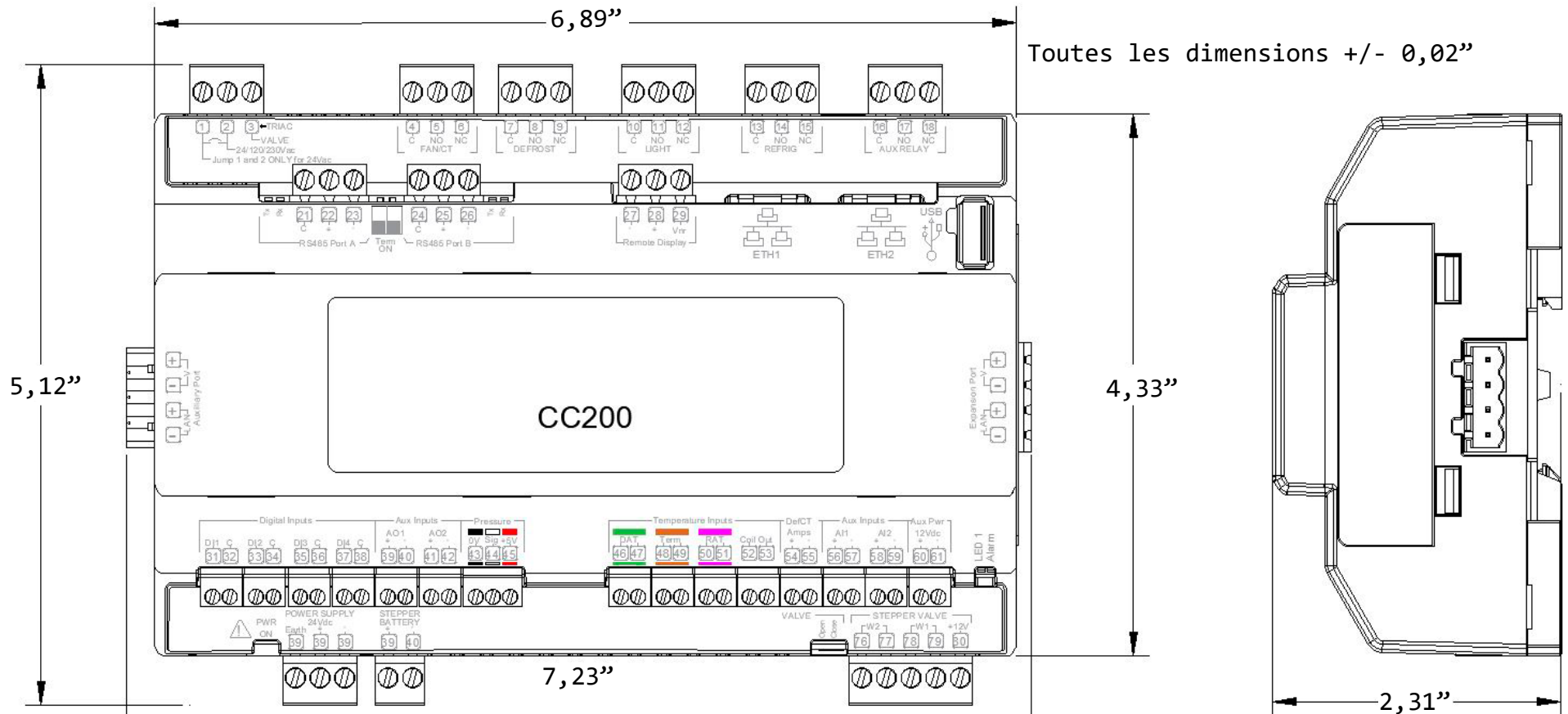
CC200 Dimensions P/N 810-3180
