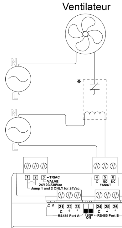
Ventilateurs alternatifs de plus de 5 ampères
