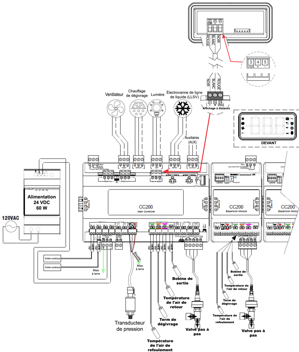
Câblage et connexions du CC200
