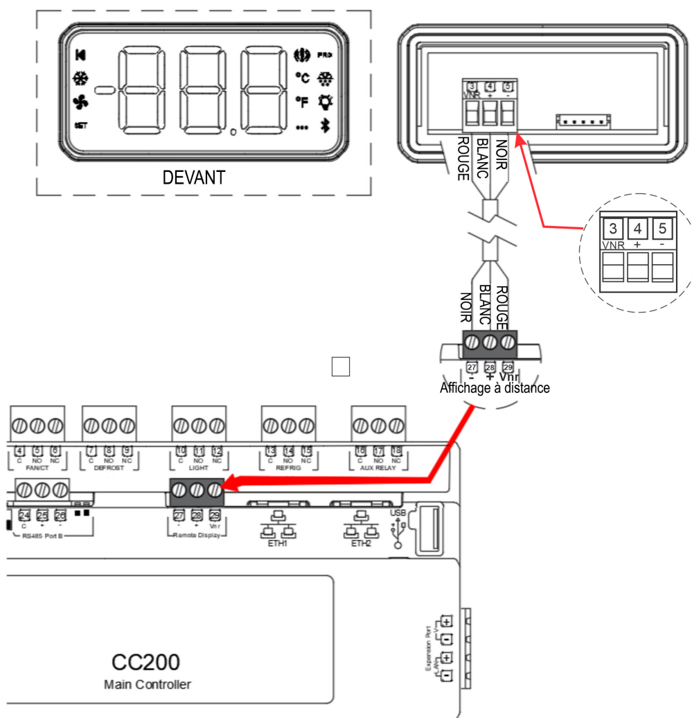
Câblage de l'affichage du boîtier CC200
