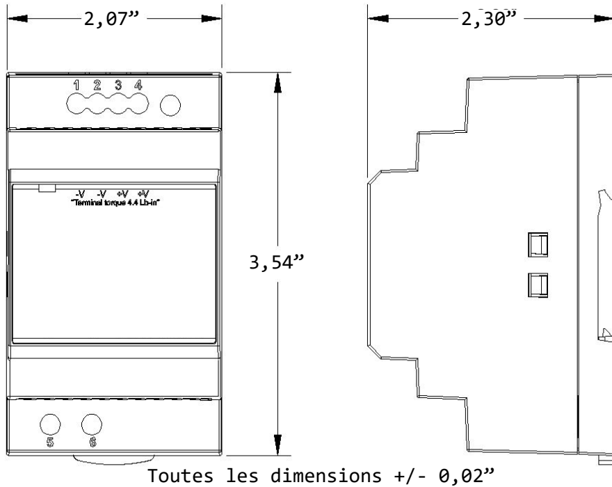
Dimensions de l'alimentation 60 watts P/N 318-3183
