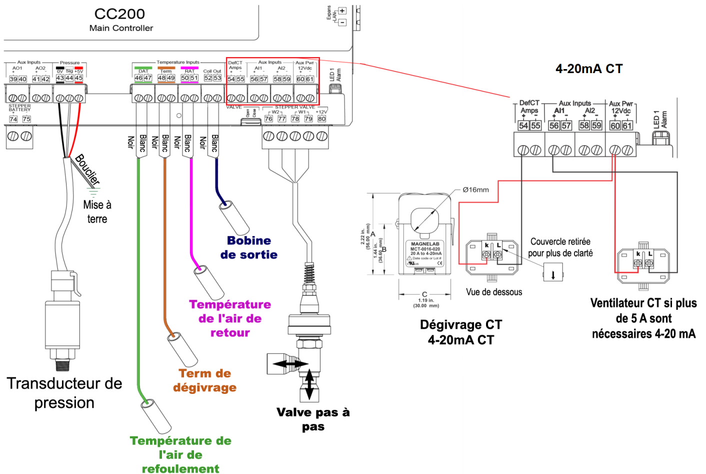
Câblage d'entrée
