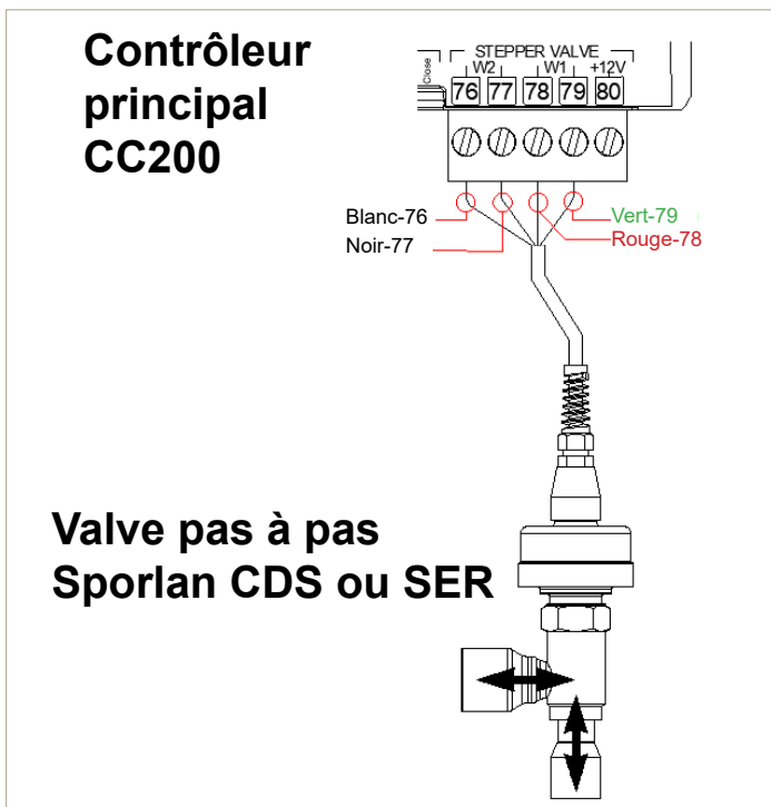
Câblage de la valve pas à pas du contrôleur principal
