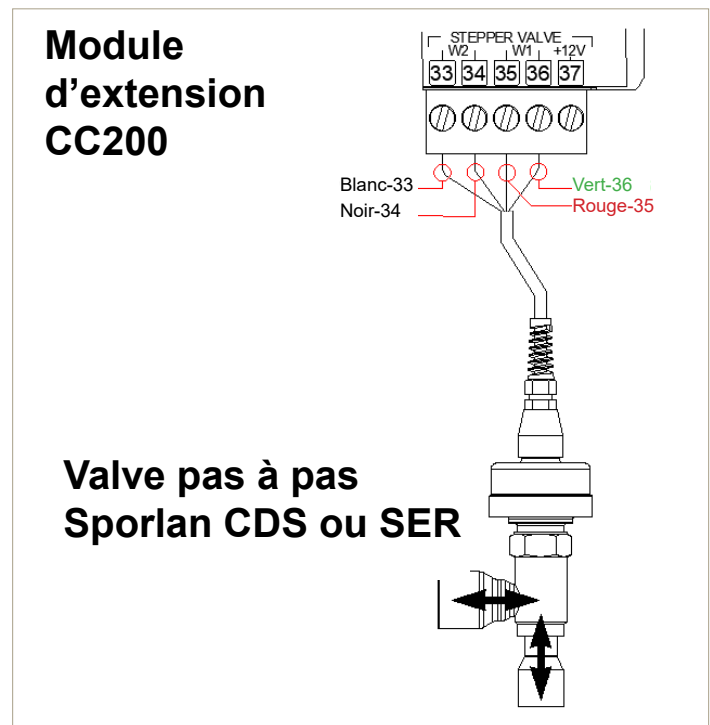
Câblage de la valve pas à pas du module d'extension
