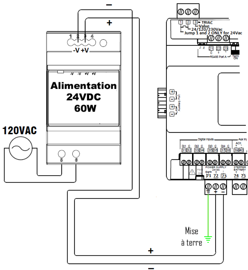
Câblage de l'alimentation CC200
