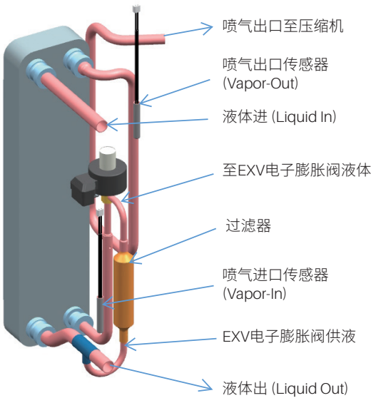
下游取液板换安装示意图
