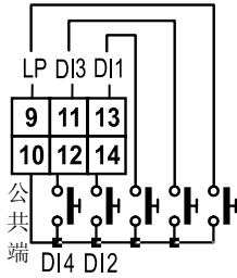
DI1-4、LP 接线
