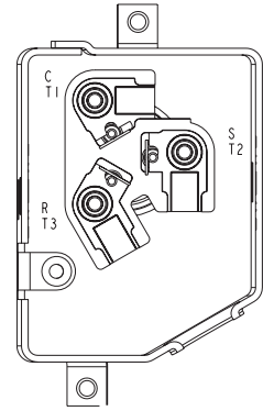
T-BOX LAYOUT OPTIONAL SCALE 3:2
