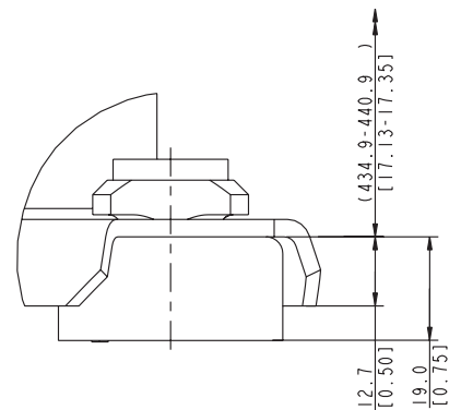
DETAIL Y SCALE 2:1
